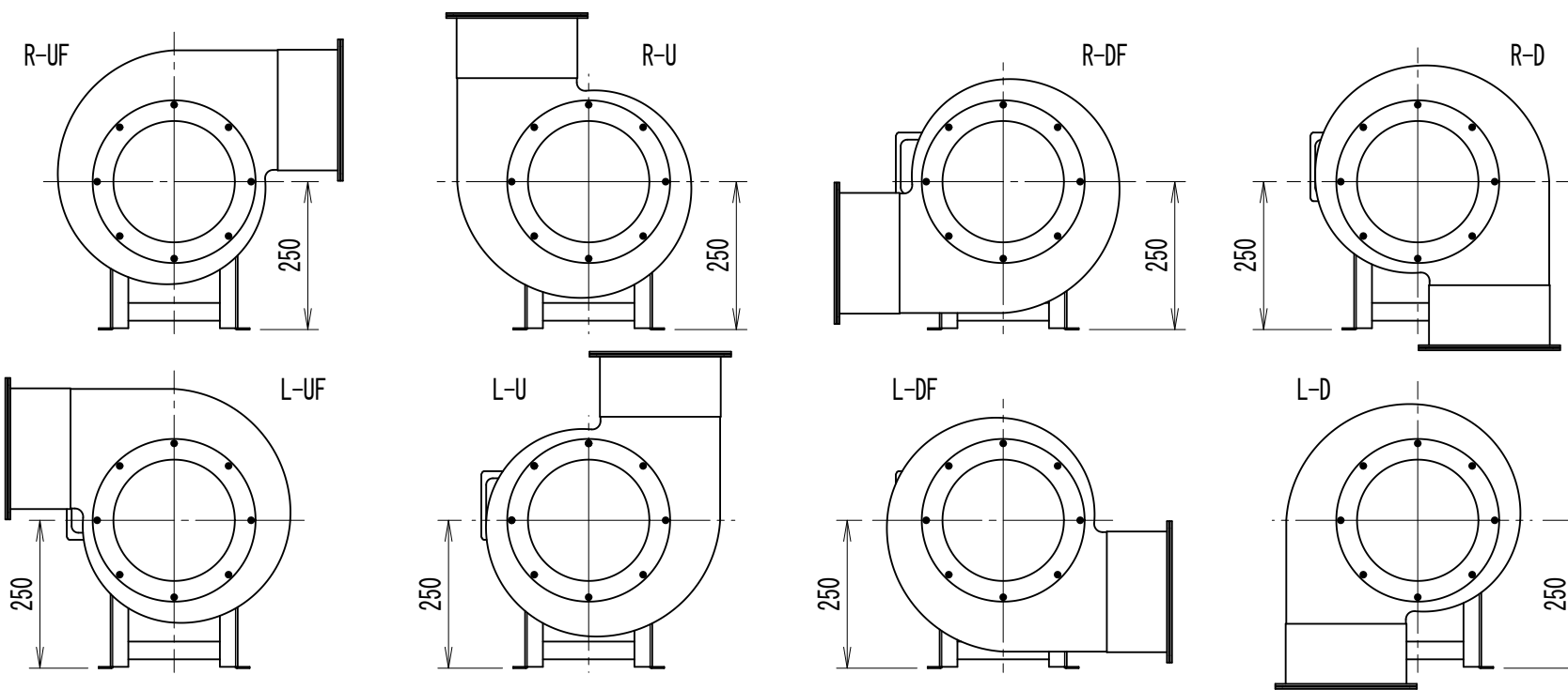
吐出方向一覧 (縮尺 1 : 1.2) 主要寸法は上図と同じになります。
